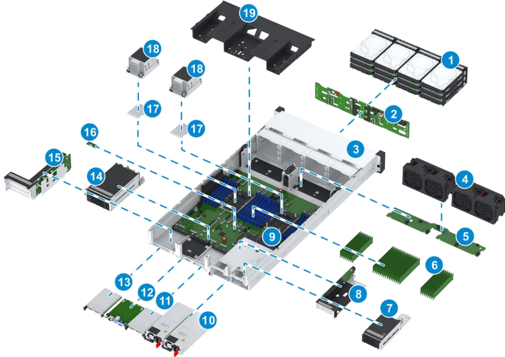
Figure 3-1 Fiziksel Yapı
