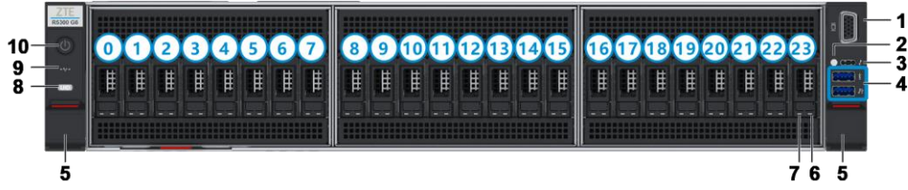
Figure 2-7 Yirmi Dört E1.S Disk Yuvalı Ön Panel
