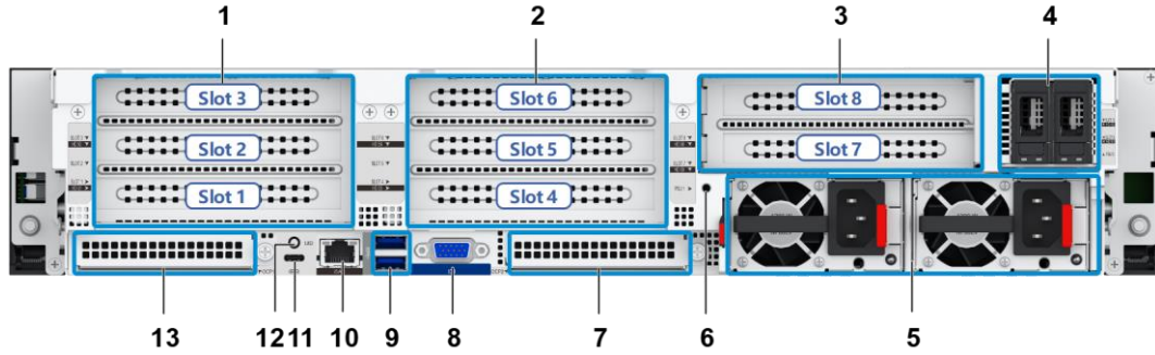
Figure 2-10 Sekiz Tam Yükseklikte PCIe Kartlı Arka Panel
