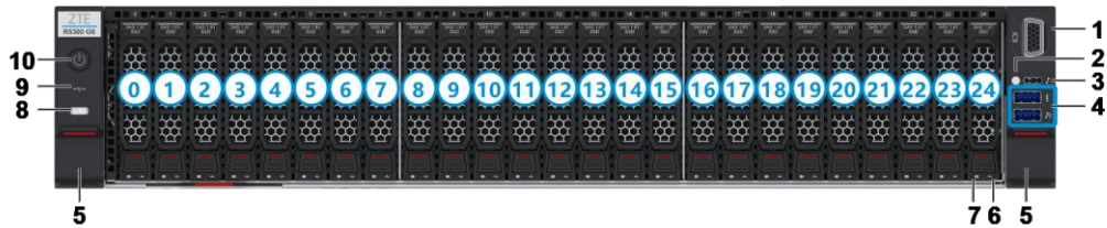
Figure 2-6 Yirmi Beş Dikey Disk Yuvalı Ön Panel
