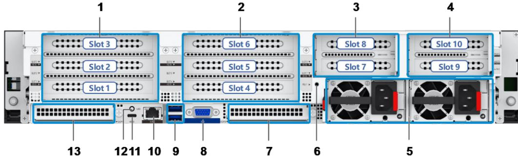
Figure 2-9 Altı Tam Yükseklikte PCIe Kartlı ve Dört Yarım Yükseklikte PCIe Kartlı Arka Panel
