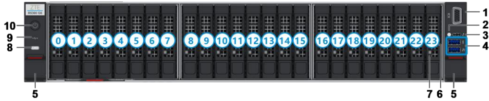
Figure 2-8 Yirmi Dört E3.S Disk Yuvalı Ön Panel
