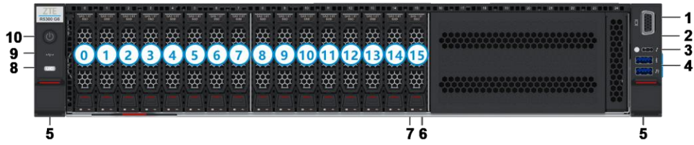
Figure 2-4 On Altı Dikey Disk Yuvalı Ön Panel
