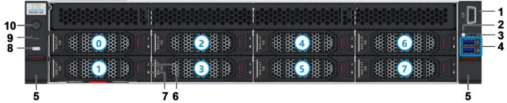
Figure 2-1 Sekiz Yatay Disk Yuvalı Ön Panel
