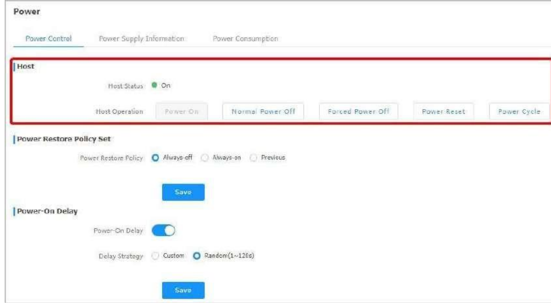
Şekil 5-9 Power Sayfası
