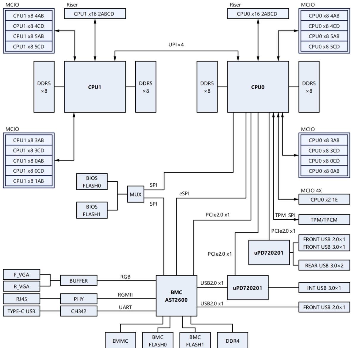
Figure 3-2 Mantıksal Yapı
